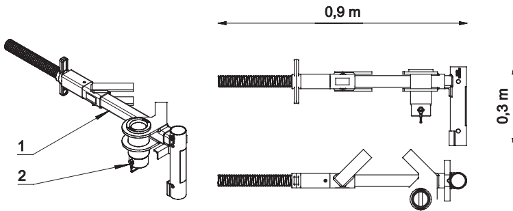
Abbildung 11. Stahlflanschzwingensatz MkII - NEU
