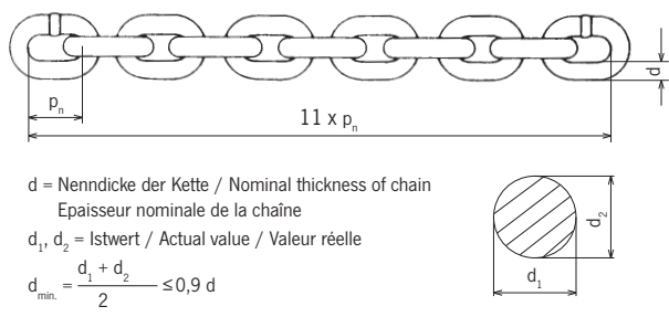
Nominalwerte und Verschleißgrenzen / Nominal values and wear limitation Valeurs nominales et limites d'usure
